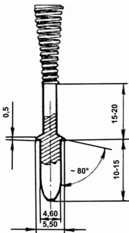
Рис. 1. Наружный калибр для определения достоинства пробоины в стрельбе из пневматической винтовки
