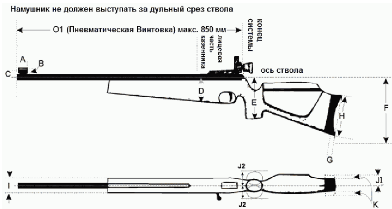
Рис. 1. Размеры стандартной пневматической винтовки.
