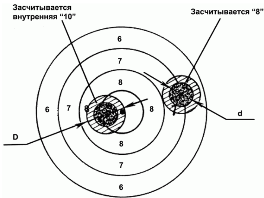
Рис. 2. Примеры использования шаблона
