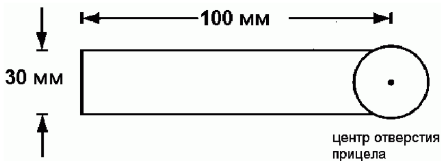
Рис. 1. Затемнитель для глаза
